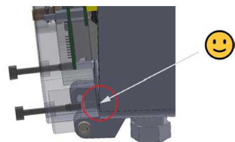
Abb. 23-4 Verschlusschrauben: gesichert / Kollision vermieden
