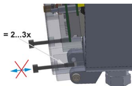
Abb. 23-4 Verschlusschrauben: gesichert / Kollision vermieden
