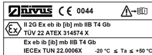
Abb. 18-2 Typenschild (Teil 2, nur bei Ex-Geräten) NivuLink Micro II Ex
