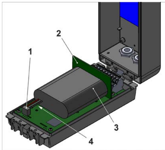
Abb. 48-2 Akkutausch
