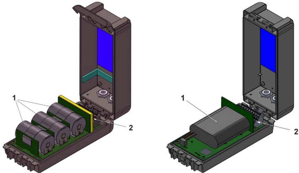
Abb. 3-1 Spannungsversorgung durch Batterien / Akku
