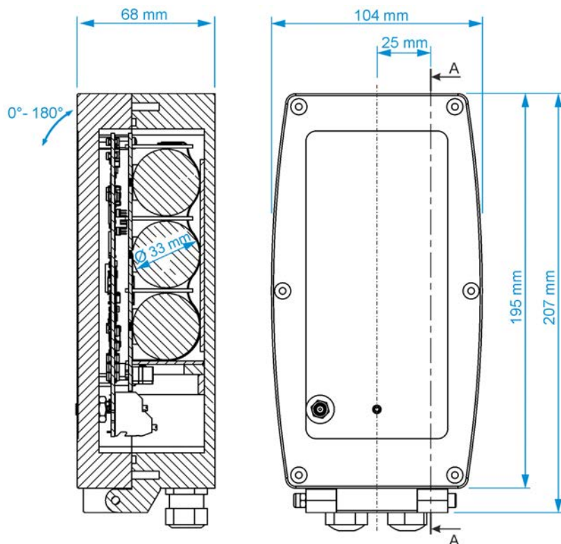
Abb. 17-5 Gehäuse für Ex Gerätevariante
