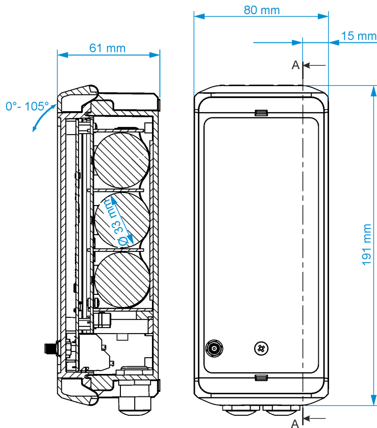
Abb. 17-4 Gehäuse für Nicht-Ex Gerätevarianten
