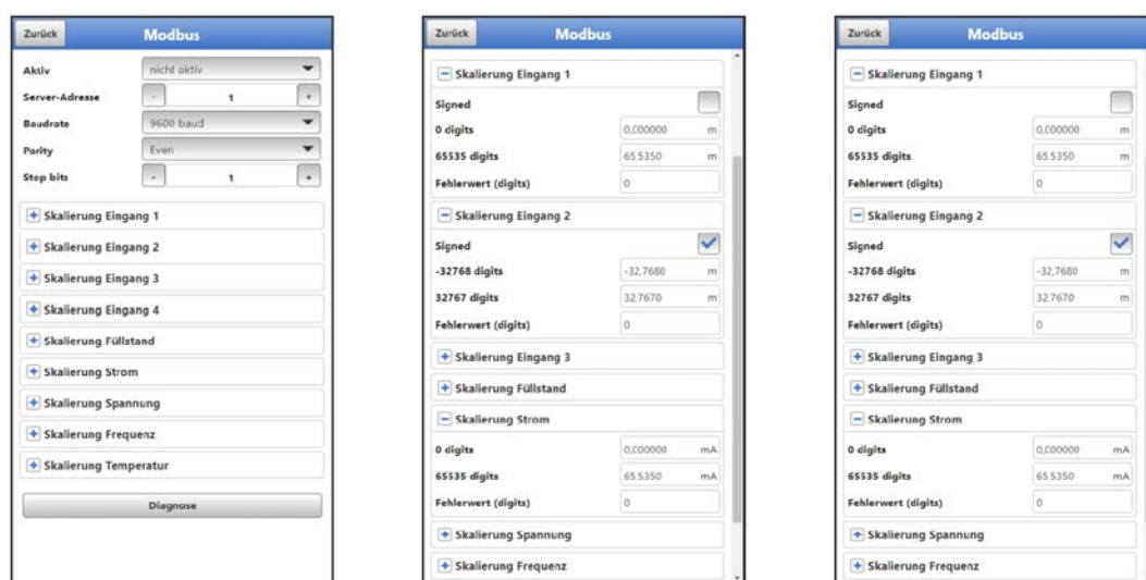
Abb. 42-8 Modbus / Skalierung
