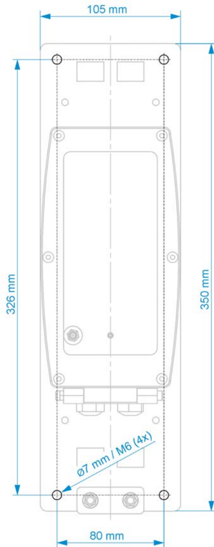
Abb. 24-1 Befestigungsbohrbilder
